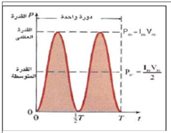
شكل 6-4 منحنى القدرة في مقاومة أومية خالصة
