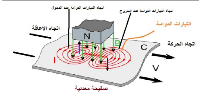
شكل 3-6 يوضح التيارات الدوامية
