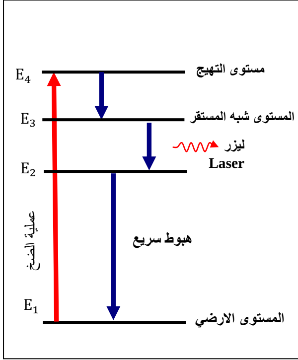
الشكل 6-15 منظومة ليزر رباعية المستوى
