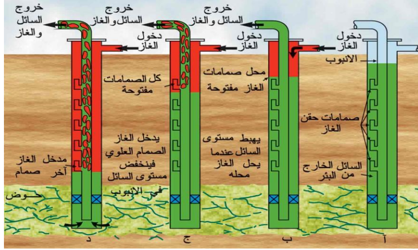
الشكل 5-7 كيفية استخراج النفط الخام
