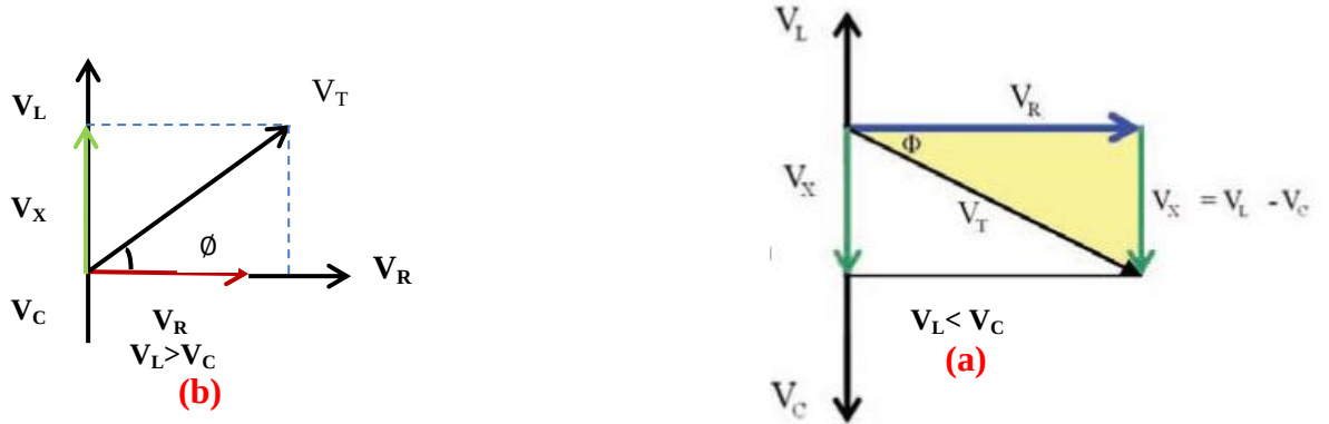
شكل 16-4 مخطط الفولتية الطوري. (a) مخطط يوضح الخواص السعوية. (b) مخطط لتوضيح الخواص الحثية يكون التيار هنا متساوي ( I_T = I_R = I_L = I_C )
