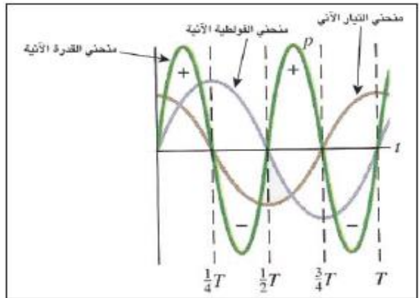
شكل 10-4 يمثل منحنى القدرة
