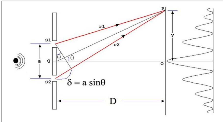
الشكل 5-2 مخطط لتجربة يونك شعاعيا
