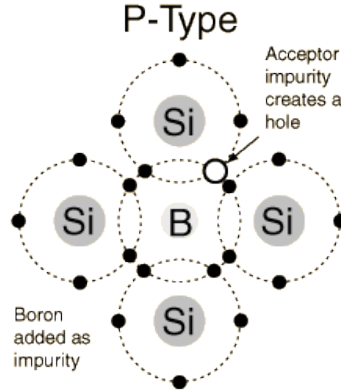
شكل 8-5 يوضح شبه الموصل من نوع الموجب
