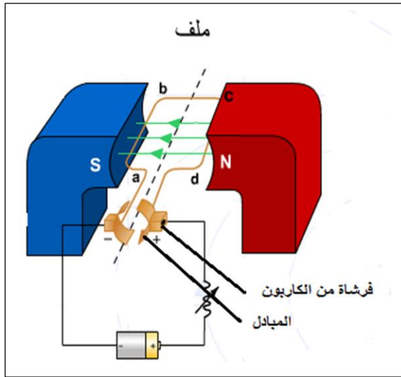
شكل 3-14 رسماً تخطيطياً لمحرك بسيط
