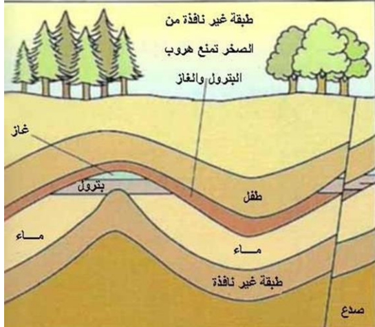
شكل 3-7 يبين وجود النفط الخام داخل قشرة الارض
