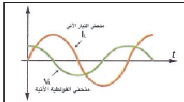
شكل 4-8-a موجة الفولتية والتيار في دائرة المحث
