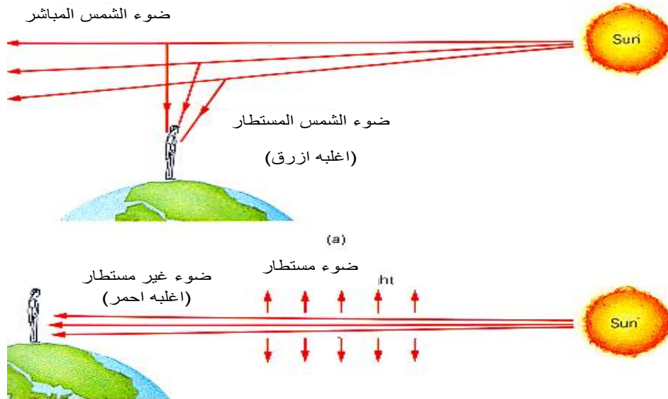
الشكل 2-15 بسبب استطارة اللون الأزرق من جزيئات الجو تحصل زرقة السماء و المتبقي من الضوء يكون أحمر و هذا يجعل لون الشمس عند الغروب و الشروق بلون أحمر.
